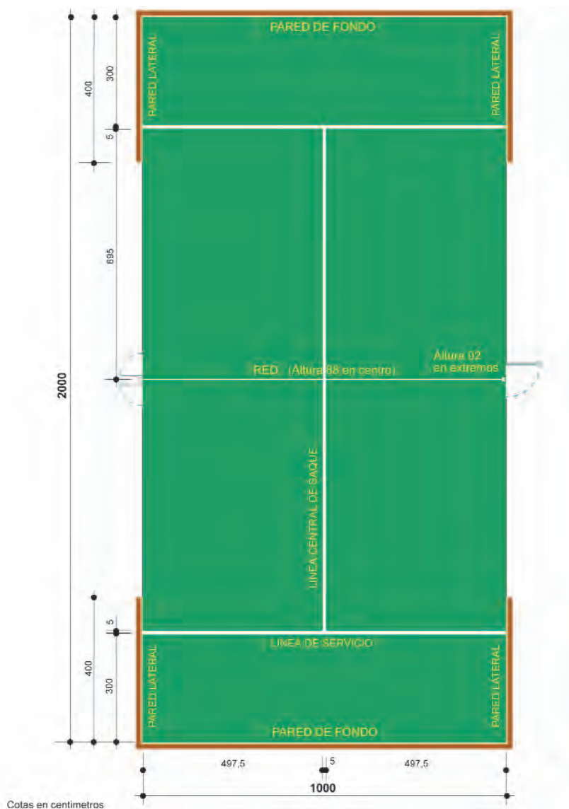
Campo de juego de pádel según normas NIDE.
