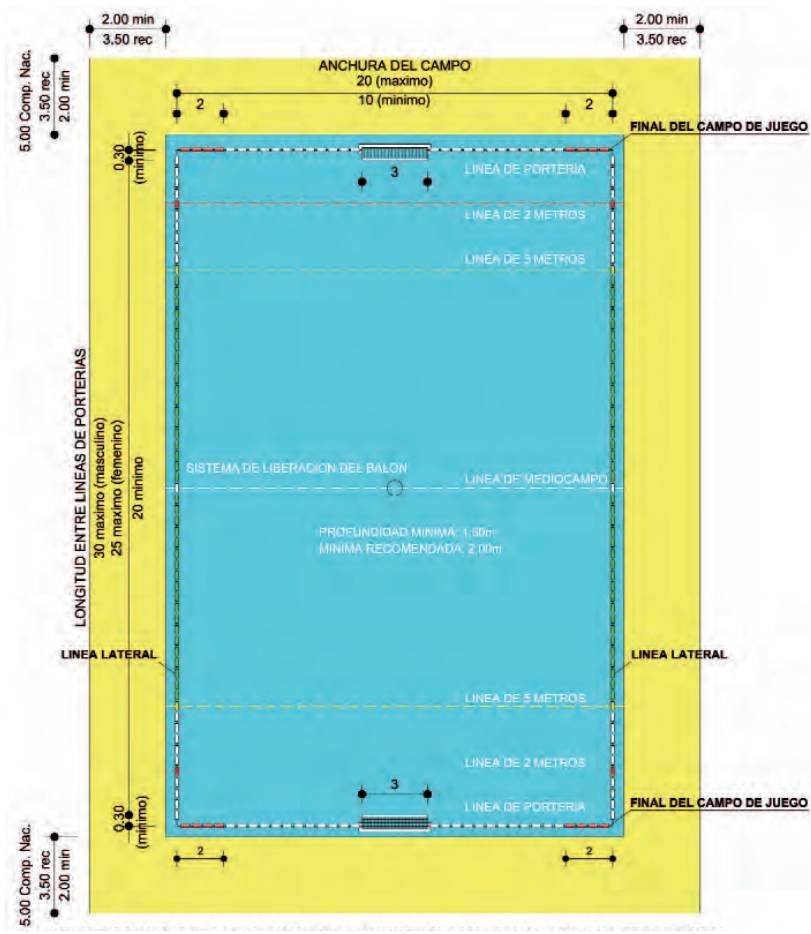
Piscina de waterpolo según normas NIDE.
