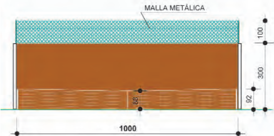
ALZADO FONDO
