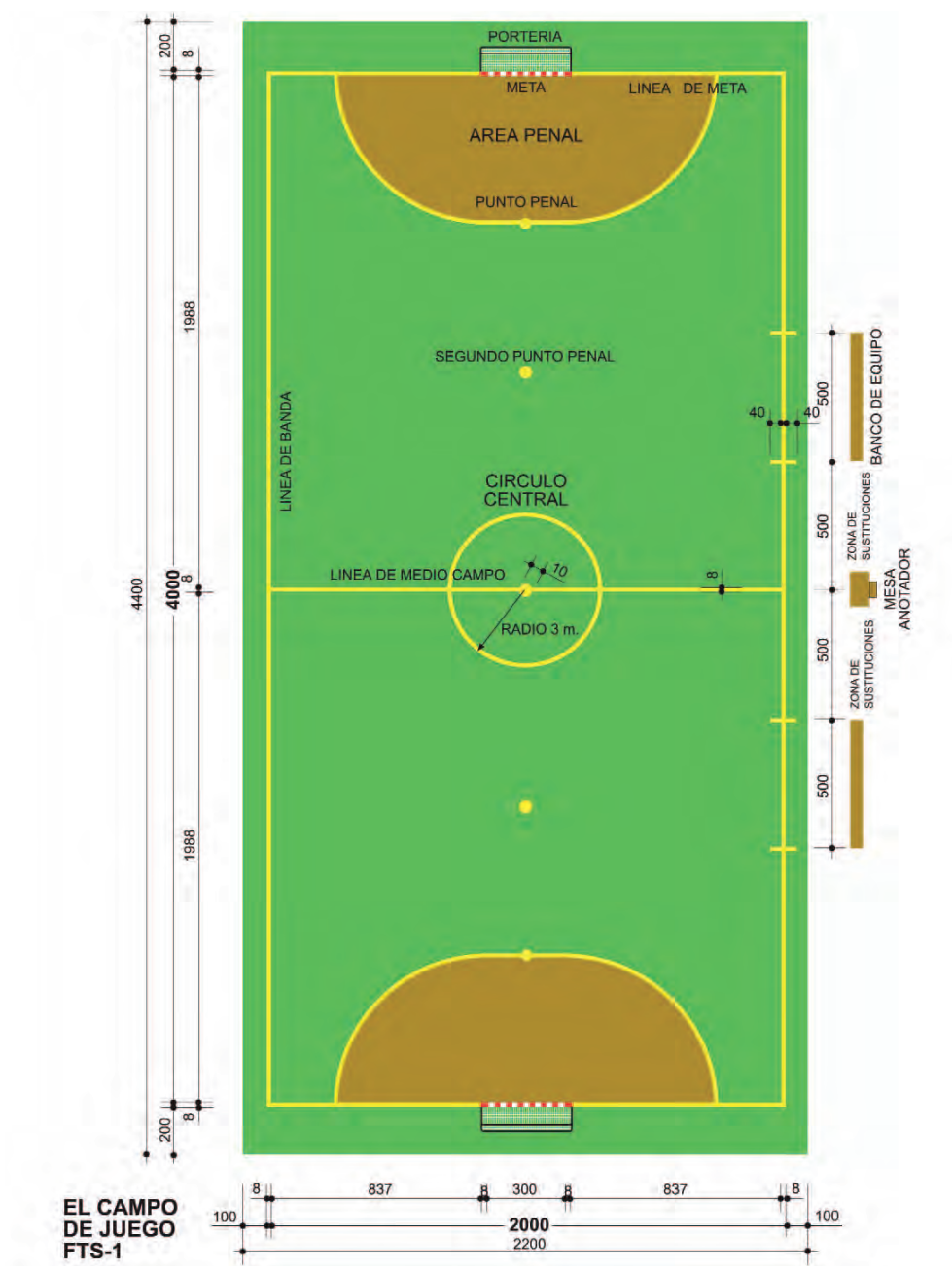
Campo de juego de fútbol sala según normas NIDE.
