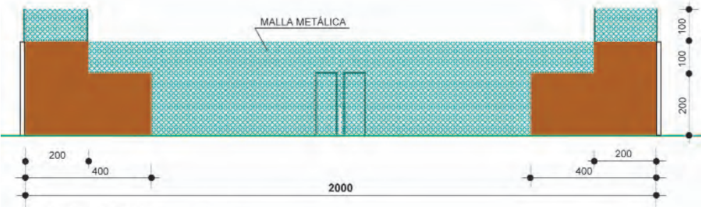
ALZADO LATERAL - variante 1
